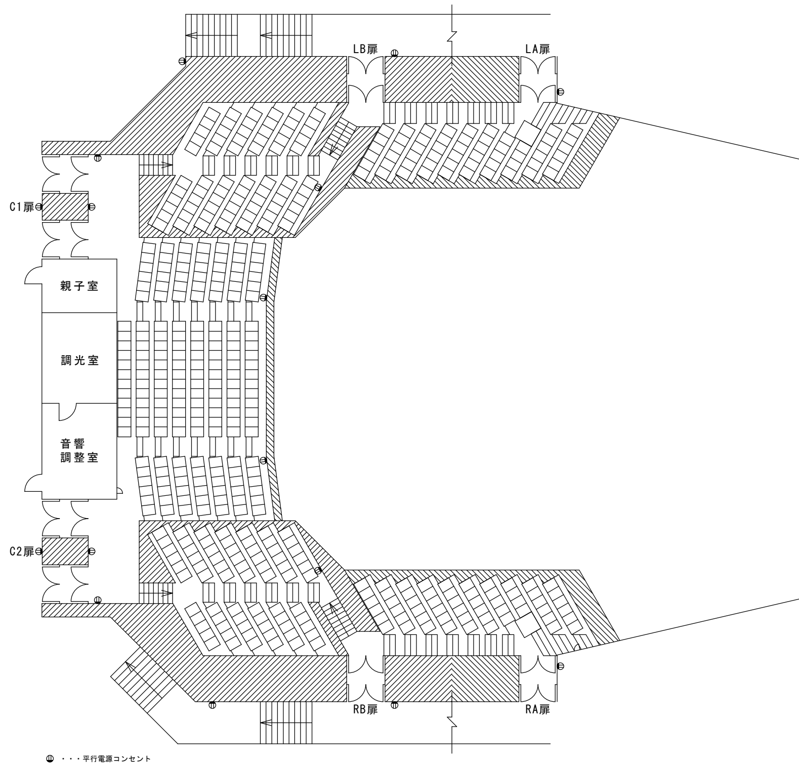
和光市民文化センター 大ホール2階平面図（音響用） A3 S=1/200
